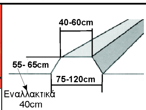
mögliche Dammmasse
