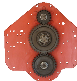
Zahnradseitentrieb
