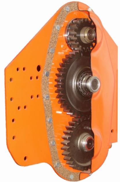
Zahnradseitentrieb
