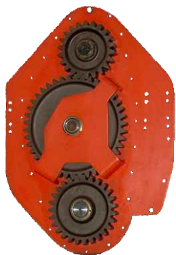
Zahnradseitentrieb
